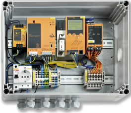
TNC-SVC02DPR (BEISPIEL)
