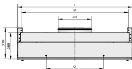
Maßzeichnung TFM
