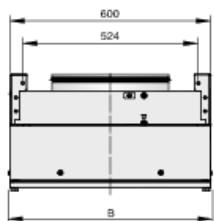
Maßzeichnung TFM
