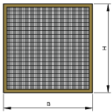
MFP-...-MDF, Seitenansicht
