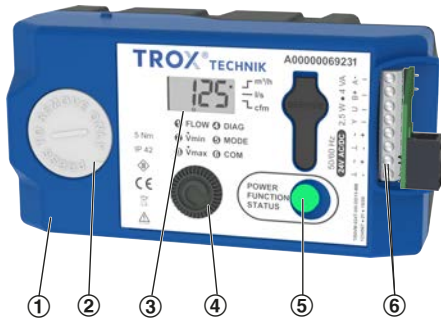
Compactregler XS0-J6 für TVE
