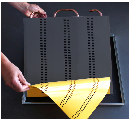
Abb. 6: Schutzfolie vom Kühlelement entfernen und somit Hochleistungsklebeband aktivieren
