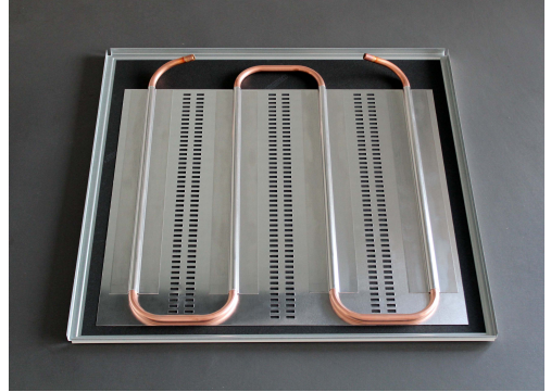
Abb. 9: Aktivierte Deckenplatte kann nun zur weiteren Montage verwendet werden
