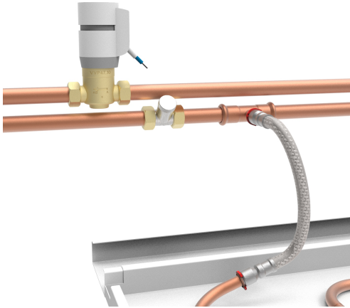
Abb. 13: Anschluss an Wasserstrang
