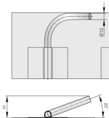
Abb. 11: Rohranschluss 90°
