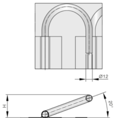
Abb. 12: Rohranschluss 180°
