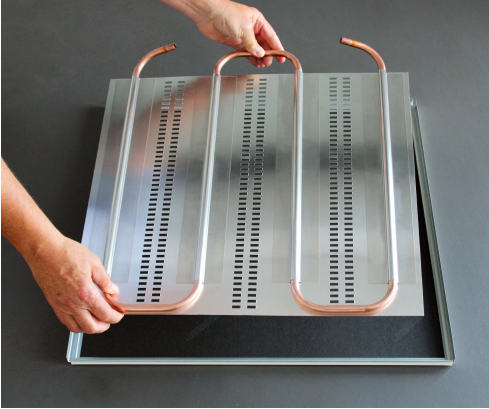
Abb. 7: Kühlelement mit der Klebefläche auf das bauseitige Deckenelement auflegen
