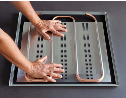
Abb. 8: Gleichmäßiges händisches Anpressen des Kühlelementes um eine dauerhafte Verbindung zur Deckenplatte zu schaffen
