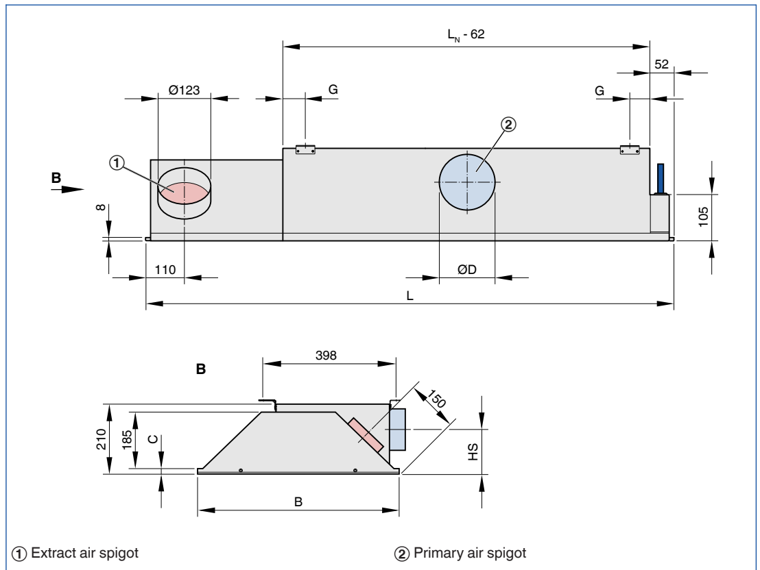
Type DID632-...-RR-AV
